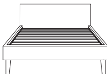
Double bed w 207 d 146 h 95
